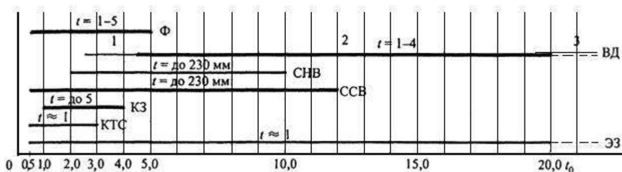
Рисунок 4.2 - Область применения различных видов СМС в зависимости от сочетания толщин соединяемых элементов
