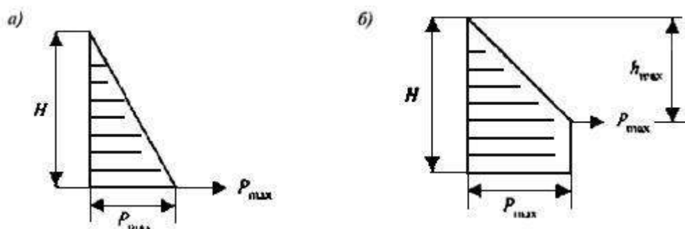
Рисунок С.1 - Расчетные эпюры бокового давления бетонной смеси
