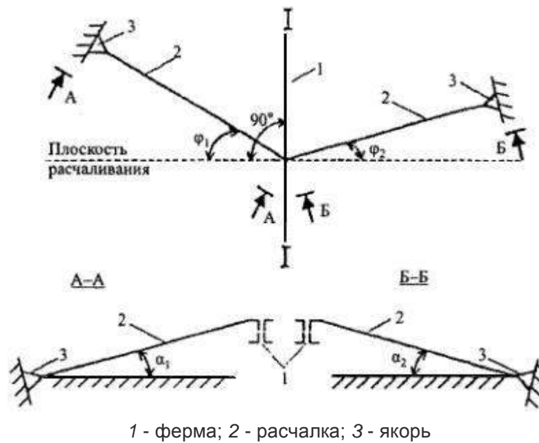
Рисунок К.2 - Схема раскрепления ферм расчалками
