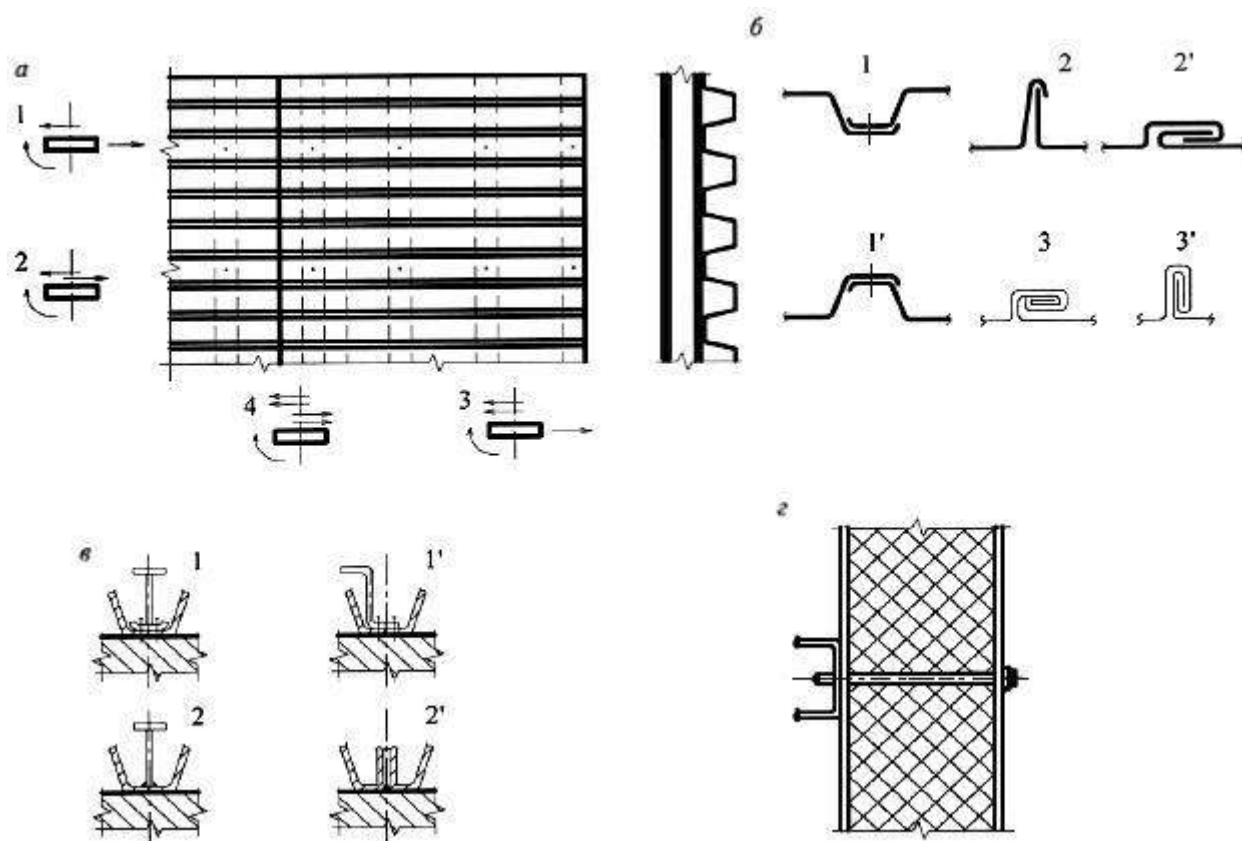
Рисунок 4.1 - Конструктивные формы СМС
